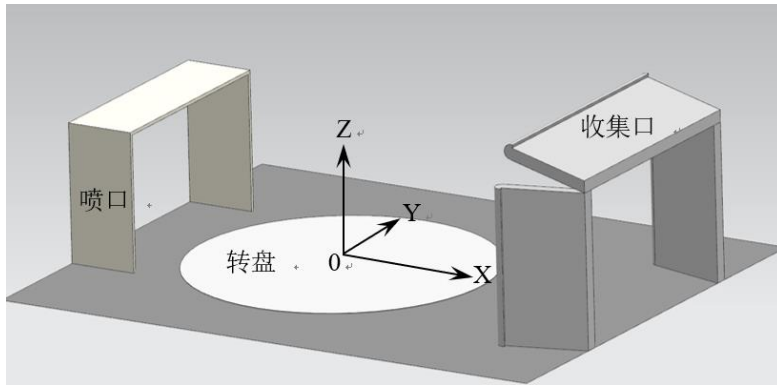
图 1 汽车空气动力学风洞坐标系
