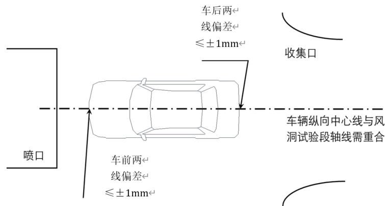
图4 车辆纵向中心线与试验段轴线重合定位示意
