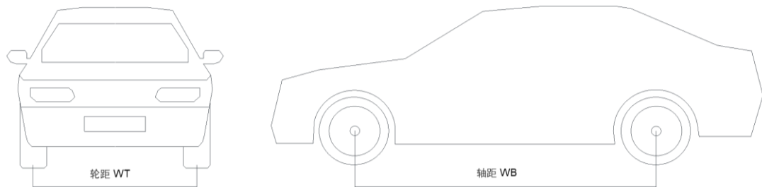
图 2 车辆轮轴距测量位置示意
